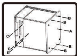
Ubicazione delle viti
